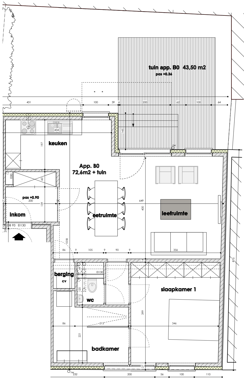
GRONDPLAN B0 1/75
